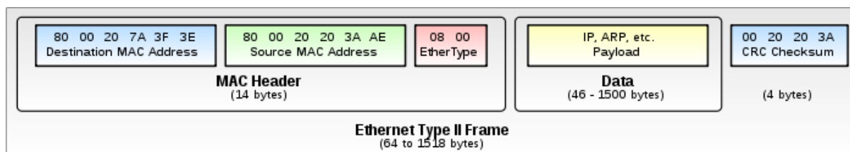
Рисунок 5.1 – Формат кадру Ethernet II
