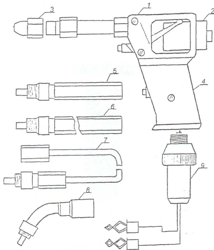
Рисунок 1 – Компресограф КБ 1126
