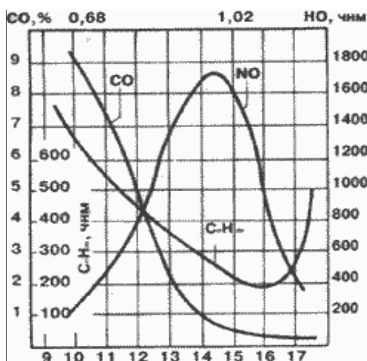
Рисунок 3 – Вміст окису вуглецю \text{CO} , вуглеводнів \text{C}_n\text{H}_m
