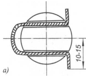
Рис. 1.1. Способи навішування свинцевих пломб з двома паралельними отворами
