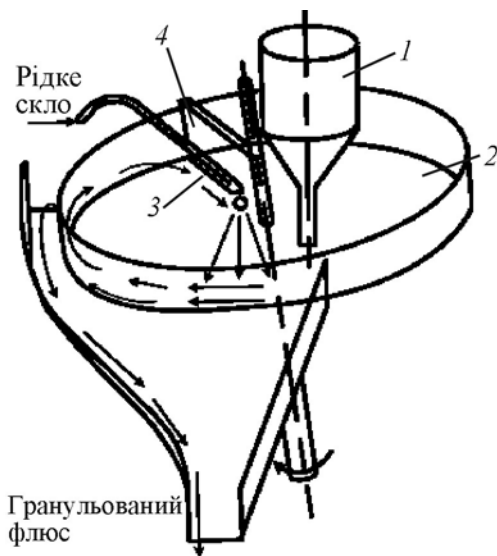
Рис. 4.5. Схема роботи дискового гранулятора
