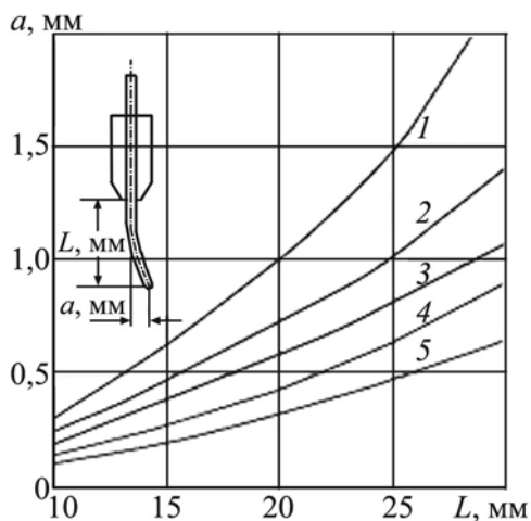
Рис. 3.2. Вплив діаметра намотування дроту d_n на коливання a кінця електрода залежно від вильоту електрода L :
