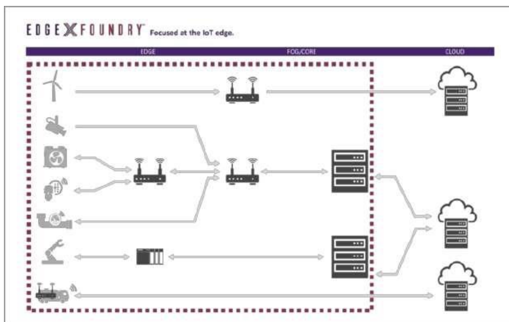
Рисунок 4.1 – Структура платформи Linux Foundation
